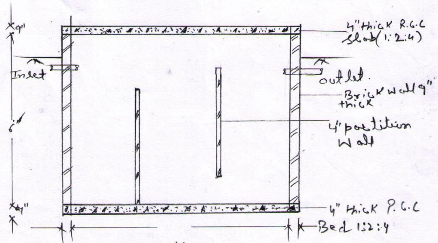
R-Section
